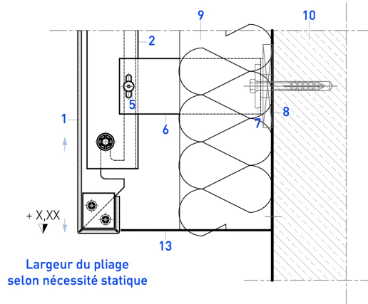
FINITION DE BAS DE FACADE (coupe verticale)
